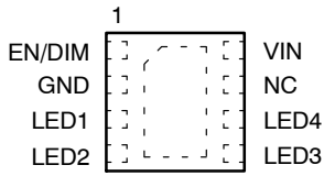
CAT4004B UDFN8 2 x 2 mm
