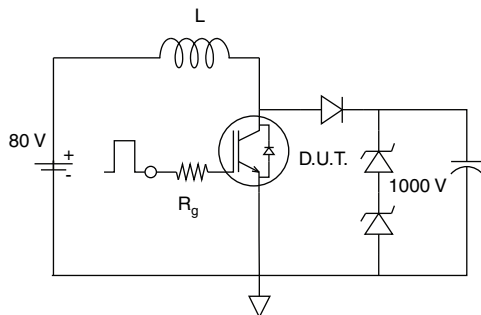
Fig. 20 - RBSOA Circuit
